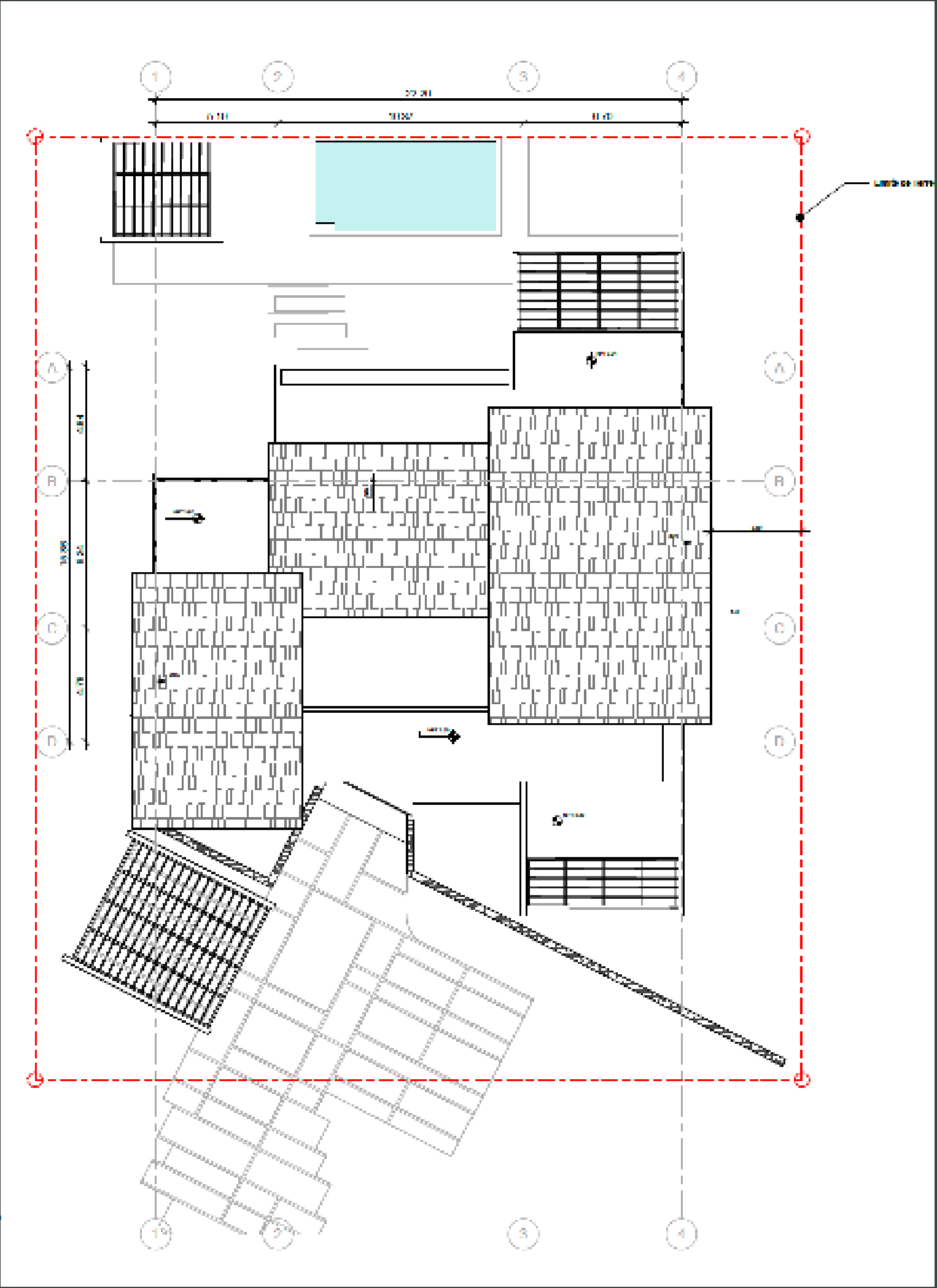
ARCHITECTURAL FLOOR ROOF PLANTA ARQUITECTÓNICA TECHO
